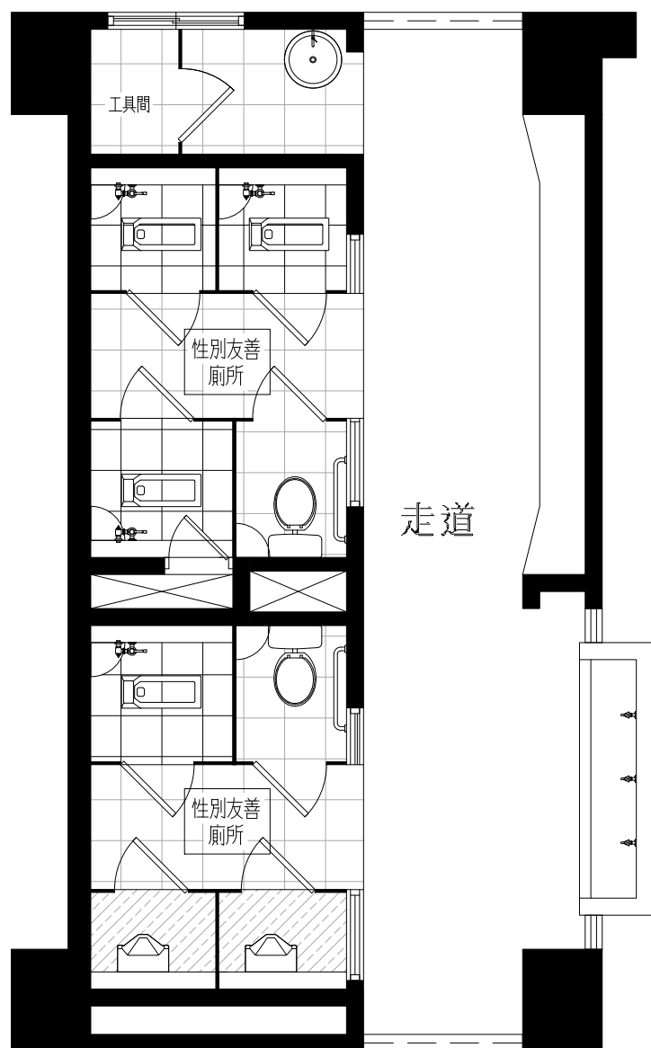
性別友善廁所平面配置圖
